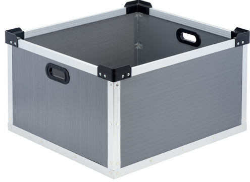
Aluminyum Çıta ve Köşebentli Tasarım / Aluminium Lath and Angle Design
