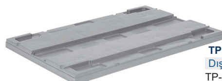
TP-65x100 En/W Boy/L Yük/H Dış / Ext 650 x 1050 x 54 mm TP-370 ve TP-400 uyumlu kapak Lid for TP-370 and TP-400
