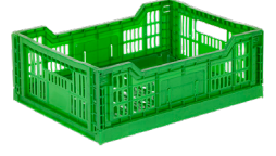
TPX-3405 En/W Boy/L Yük/H Dış / Ext 300 x 400 x 145 mm İç / Int 278 x 376 x 138 mm Katlanmış Yükseklik 30 mm Folded Height 30 mm
