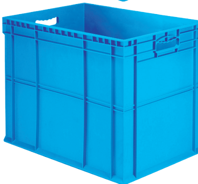
Kod / Code TP-4503 En/W Boy/L Yükseklik Dış / Ext 400 x 600 x 450 mm İç / Int 365 x 565 x 436 mm
