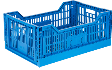
TPX-6255 En/W Boy/L Yük/H Dış / Ext 395 x 595 x 250 mm İç / Int 370 x 565 x 190 mm Katlanmış Yükseklik 55 mm Folded Height 55 mm
