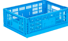
TPX-3401 En/W Boy/L Yük/H Dış / Ext 300 x 400 x 145 mm İç / Int 278 x 376 x 138 mm Katlanmış Yükseklik 30 mm Folded Height 30 mm
