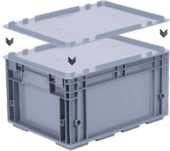
TP-30X40 En/W Boy/L Yük/H Dış / Ext 300 x 400 x 10 mm 300 X 400 mm R-KLT & RL-KLT Kullanılır / Used with
