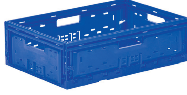
TP-6418 En/W Boy/L Yük/H Dış / Ext 400 x 600 x 177 mm İç / Int 372 x 573 x 173 mm Katlanmış Yükseklik 32 mm Folded Height 32 mm
