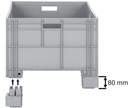
Kod / Code TP-86 AYK En/W Boy/L Yük/H Dış / Ext 60 x 50 x 80 mm TP-8650 ve TP-8639 uyumlu 80 mm yükseltme takozu, transpalet ve forkliftle kullanılmasını sağlar. 80 mm rising wedges are compatible with TP-8650 and TP-8639 and are used to make crates compatible with transpallet and forklift
