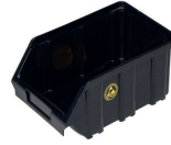
A-100-ESD En/W Boy/L Yük/H Dış / Ext 102 x 170 x 74 mm
