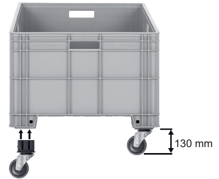
Kod / Code TP-86-T En/W Boy/L Yük/H Dış / Ext 60 x 50 x 130 mm TP-8650 ve TP-8639 uyumlu teker. Compatible wheels for TP-8650 and TP-8639
