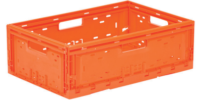
TP-6420 En/W Boy/L Yük/H Dış / Ext 400 x 600 x 197 mm İç / Int 372 x 573 x 193 mm Katlanmış Yükseklik 32 mm Folded Height 32 mm
