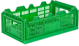
TPX-5405 En/W Boy/L Yük/H Dış / Ext 300 x 495 x 185 mm İç / Int 277 x 475 x 150 mm Katlanmış Yükseklik 30 mm Folded Height 30 mm
