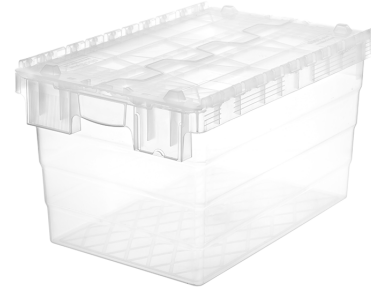
TP-6435-MK SF En/W Boy/L Yükseklik Dış / Ext 400 x 600 x 360 mm İç / Int 365 x 545 x 347 mm
