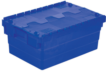
TP-6425-MK En/W Boy/L Yükseklik Dış / Ext 400 x 600 x 250 mm İç / Int 365 x 543 x 232 mm
