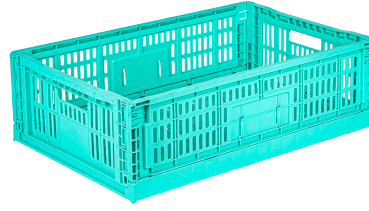
TPX-6401 En/W Boy/L Yük/H Dış / Ext 395 x 595 x 185 mm İç / Int 370 x 565 x 153 mm Katlanmış Yükseklik 55 mm Folded Height 55 mm
