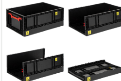
TP-4622-ESD En/W Boy/L Yük/H Dış / Ext 400 x 600 x 230 mm İç / Int 365 x 560 x 220 mm Katlanmış yükseklik 73 mm
