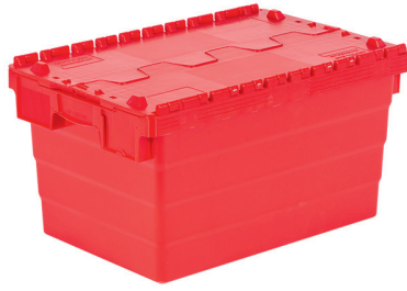
TP-6432-MK En/W Boy/L Yükseklik Dış / Ext 400 x 600 x 320 mm İç / Int 365 x 545 x 302 mm
