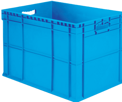
Kod / Code TP-4203 En/W Boy/L Yükseklik Dış / Ext 400 x 600 x 425 mm İç / Int 365 x 565 x 410 mm
