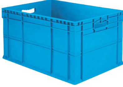
Kod / Code TP-3403 En/W Boy/L Yükseklik Dış / Ext 400 x 600 x 340 mm İç / Int 365 x 565 x 324 mm
