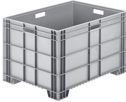
Kod / Code TP-8650 En/W Boy/L Yük/H Dış / Ext 600 x 800 x 500 mm İç / Int 565 x 760 x 435 mm
