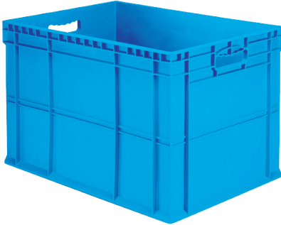
Kod / Code TP-4003 En/W Boy/L Yükseklik Dış / Ext 400 x 600 x 400 mm İç / Int 365 x 565 x 386 mm
