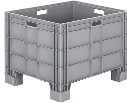
Kod / Code TP-8650-X En/W Boy/L Yük/H Dış / Ext 600 x 800 x 580 mm İç / Int 565 x 760 x 435 mm
