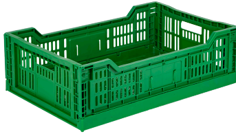
TPX-6405 En/W Boy/L Yük/H Dış / Ext 395 x 595 x 185 mm İç / Int 370 x 565 x 153 mm Katlanmış Yükseklik 32 mm Folded Height 32 mm
