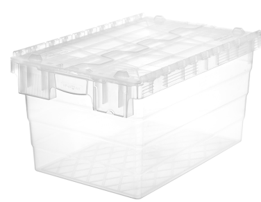
TP-6432-MK SF En/W Boy/L Yükseklik Dış / Ext 400 x 600 x 320 mm İç / Int 365 x 545 x 302 mm
