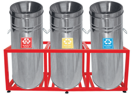
TK-1811 3'lü Atık Kovası / Metal waste bins set En/W Boy/L Yük/H Dış / Ext 1230 x 420 x 1050 mm
